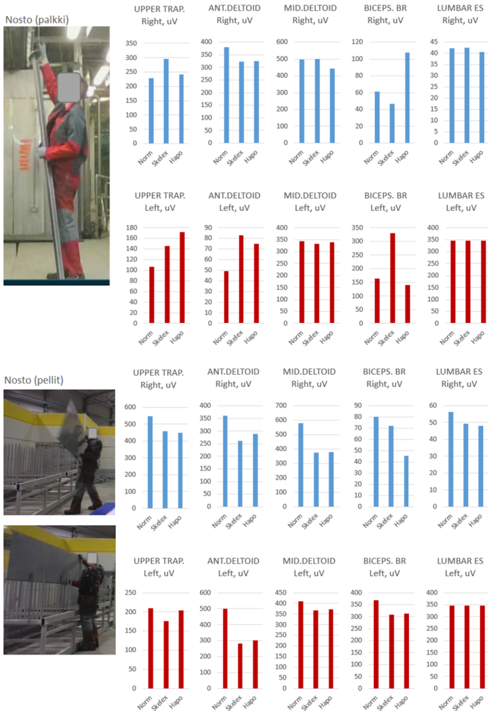
Kuva 12. Koehenkilö 2. Tutkittujen lihasten absoluuttiset EMG-tulokset normaalitilanteessa ja eksoskeleto-neilla kahdessa työtehtävässä.
