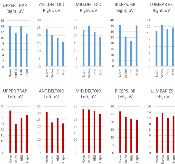
Kuva 15. Koehenkilö 6. Tutkittujen lihasten absoluuttiset EMG-tulokset normaalitilanteessa ja eksoskeletoneilla yhdessä työtehtävässä.
