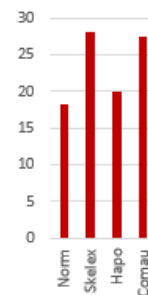
Kuva 13. Koehenkilö 3. Tutkittujen lihasten absoluuttiset EMG-tulokset normaalitilanteessa ja eksoskeletoneilla kahdessa työtehtävässä.
