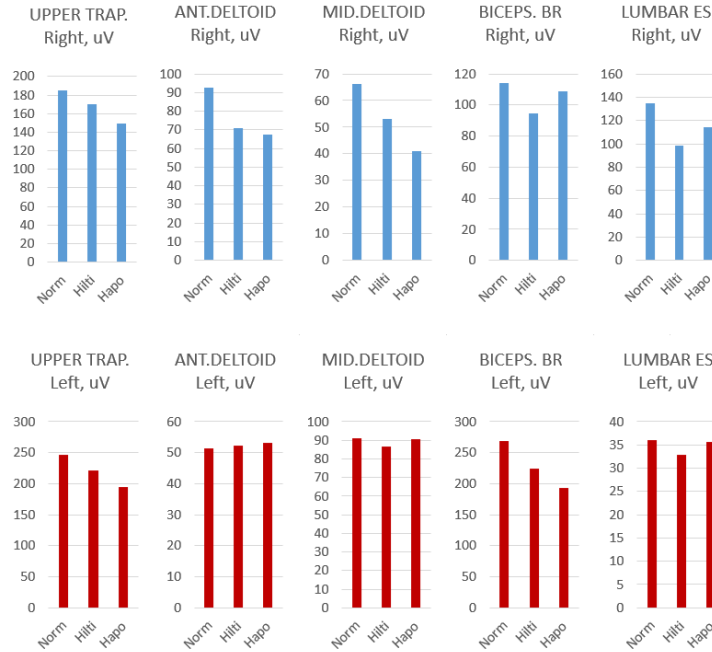
Kuva 14. Koehenkilö 4. Tutkittujen lihasten absoluuttiset EMG-tulokset normaalitilanteessa ja eksoskeletoneilla yhdessä työtehtävässä.
